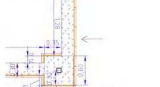
Поздовжній розріз бетонного фундаменту підріної стінки 2-3
